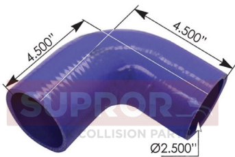
MANGUERA RADIADOR INFERIOR
