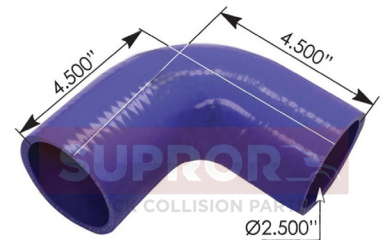
MANGUERA RADIADOR INFERIOR
