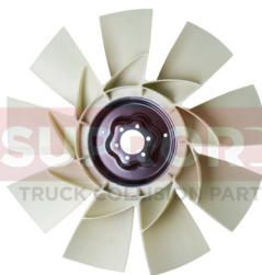
VENTILADOR 28" x 9" x 2.5" PLATO ESTRELLA
