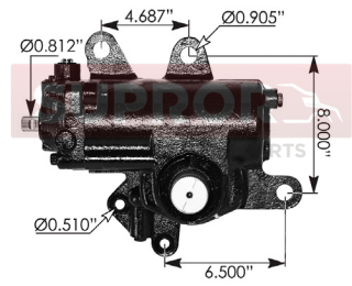
CAJA DIRECCIÓN
