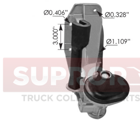
GUÍA COFRE COMPLETA R
