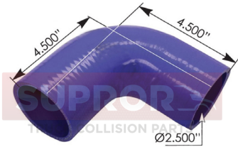
MANGUERA RADIADOR INFERIOR
