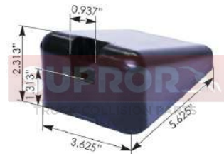
ASIENTO COFRE
