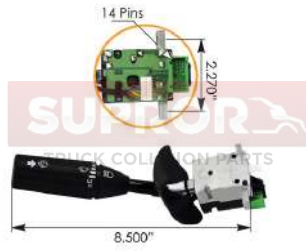
PALANCA DIRECCIONAL
